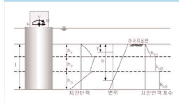
■ 그림 2. 우물통기초의 수평지반반력 분포
