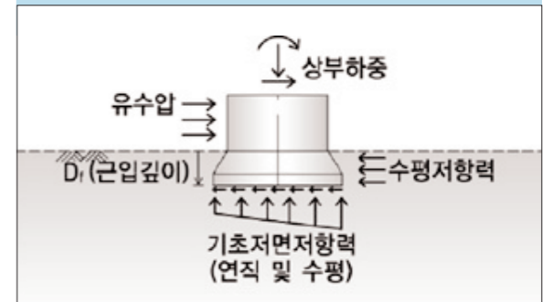
■ 그림 1. 우물통기초의 하중전달 개념도
